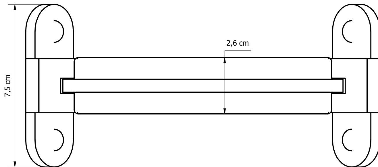
Draufsicht M -1:1-
