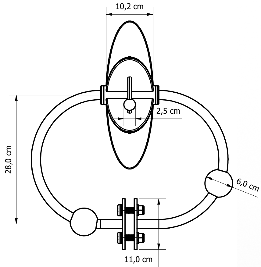
Ansicht M -1:5-
