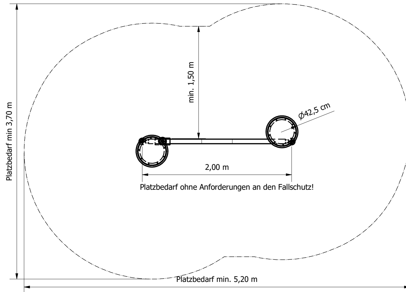
Draufsicht M -1:25-
