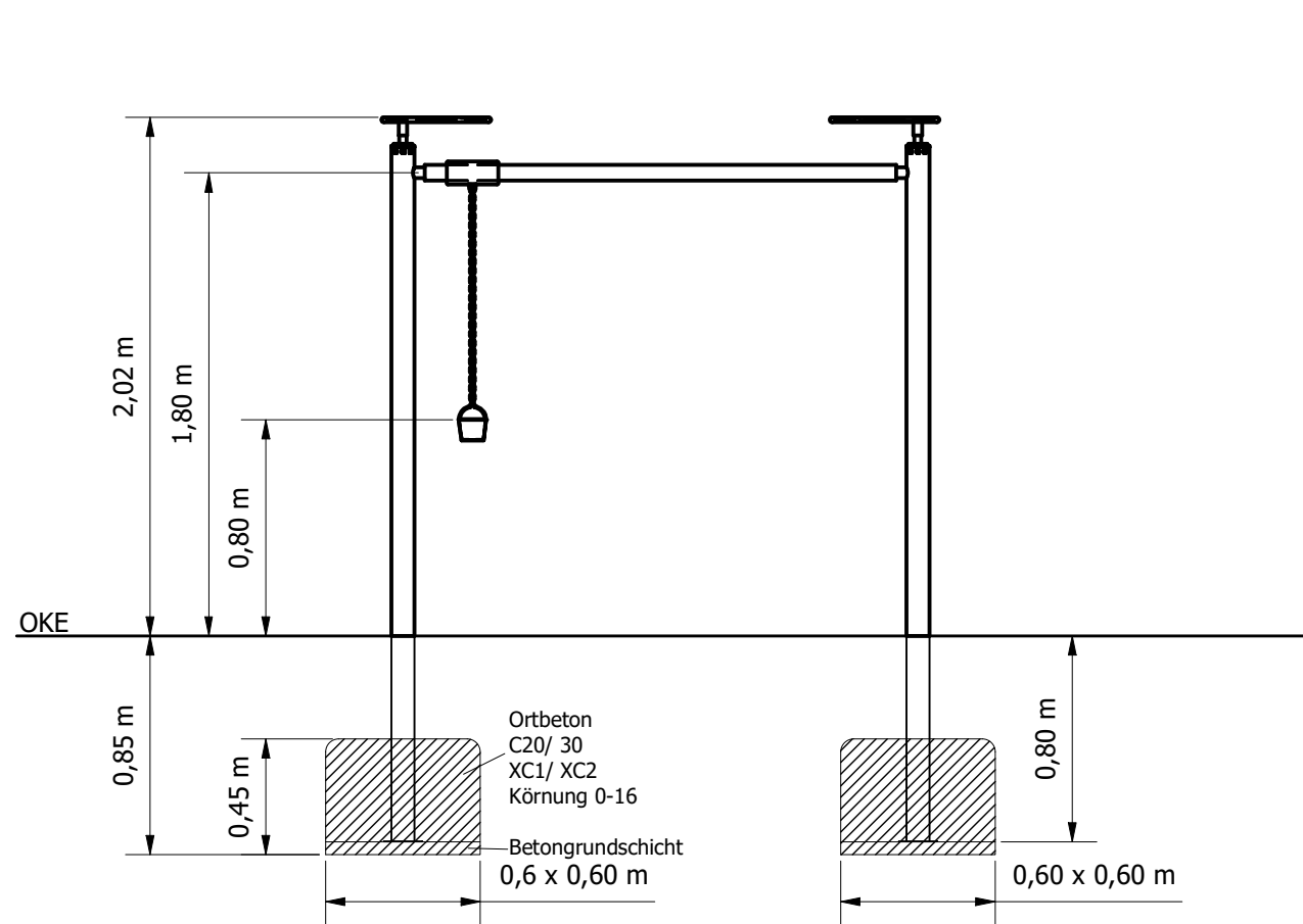
Ansicht M -1:25-
