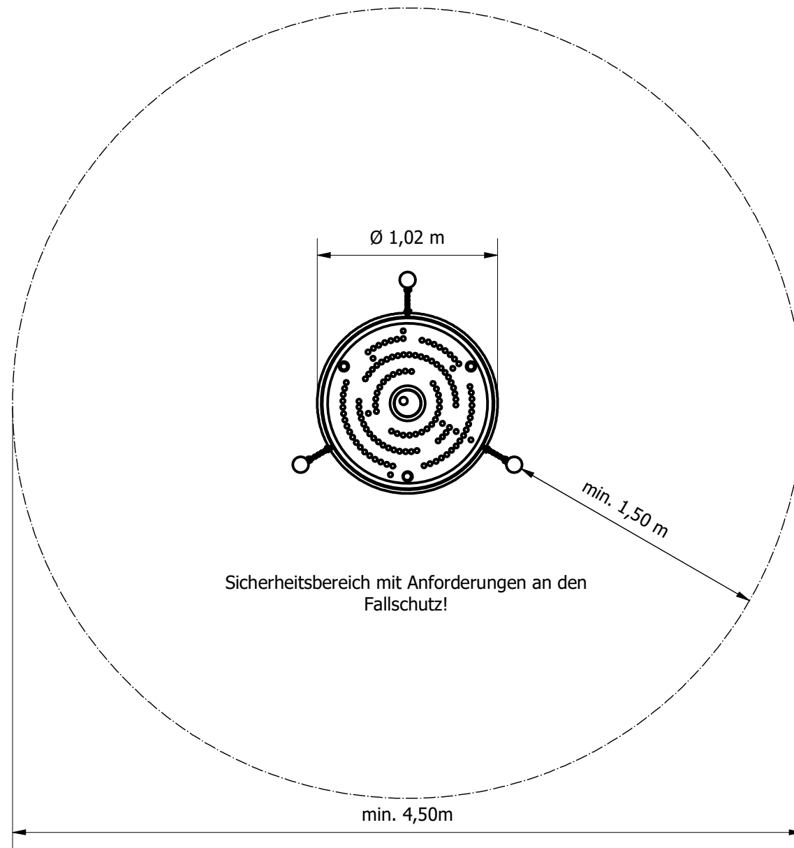
Draufsicht M - 1:25-
