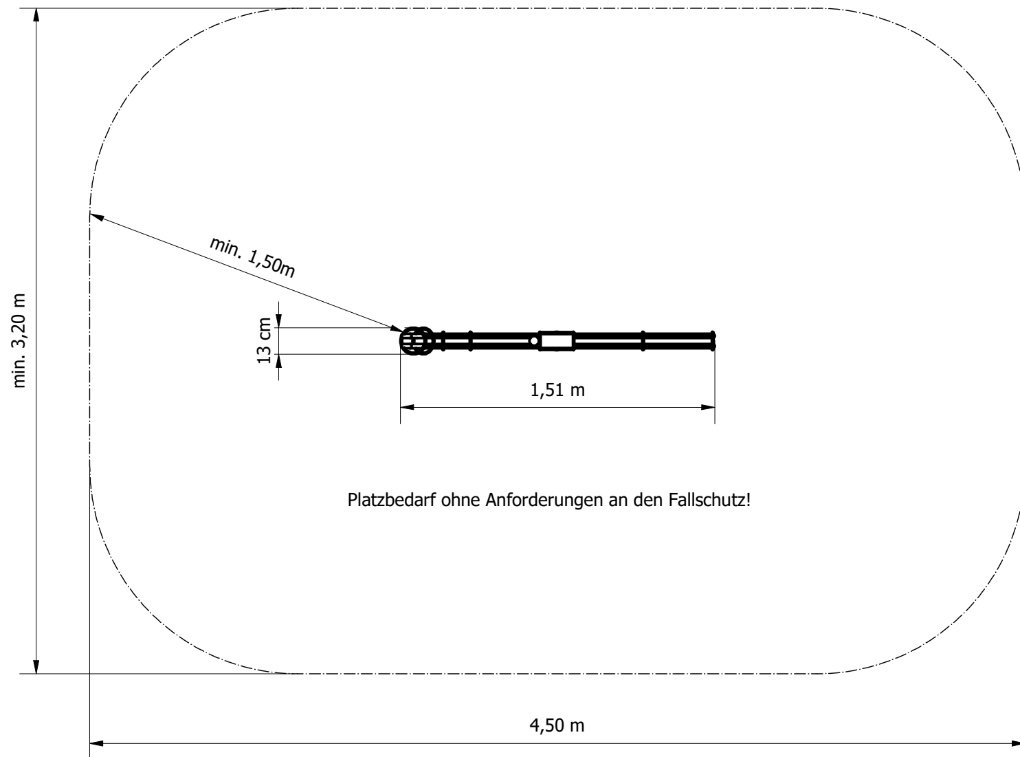
Draufsicht M - 1:25-
